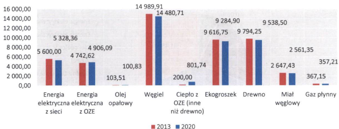
Wykres 11. Zmiana zużycia energii finalnej w perspektywie 2013-2020 – mieszkalnictwo
